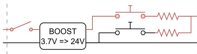
FIGURE 5.6 – Zoom sur le circuit de charge/décharge des condensateurs
