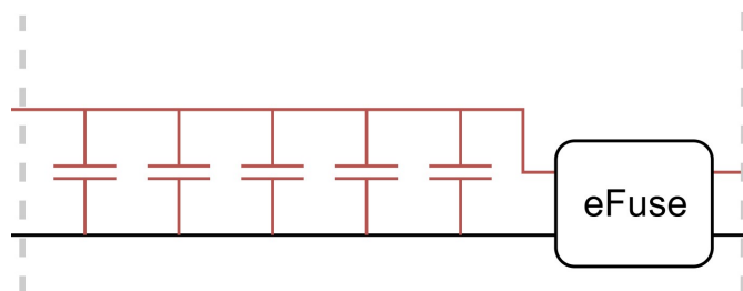
FIGURE 5.7 – Zoom sur le circuit de condensateurs
