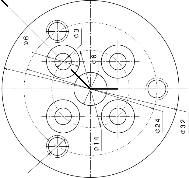
Front view Scale: 4:1
