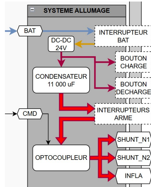
FIGURE 5.4 – Zoom sur le synopsis de la ligne de mise à feu (ref. annexe A)
