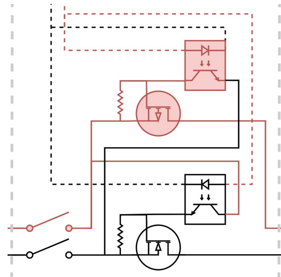
FIGURE 5.9 – Zoom sur le circuit isolateur
