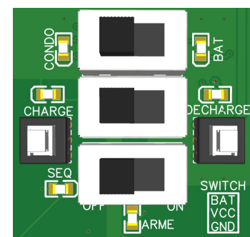
FIGURE 5.11 – Zoom sur l'interface de la carte principale du système d'allumage
