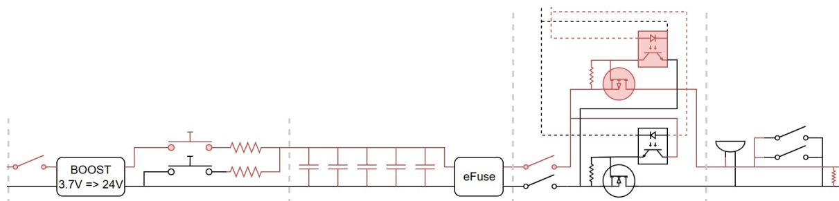
FIGURE 5.5 – Schéma de la ligne de mise à feu
