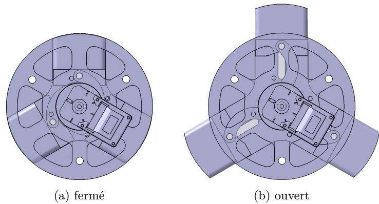
FIGURE 4.6 – Position des aérofreins d'SP-02
