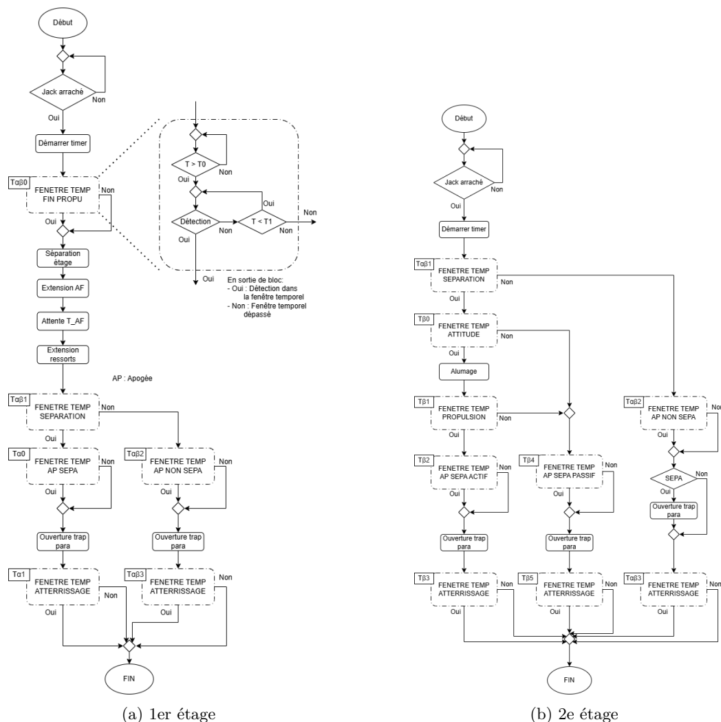
FIGURE 5.2 – Schémas fonctionnels des séquenceurs des deux étages
